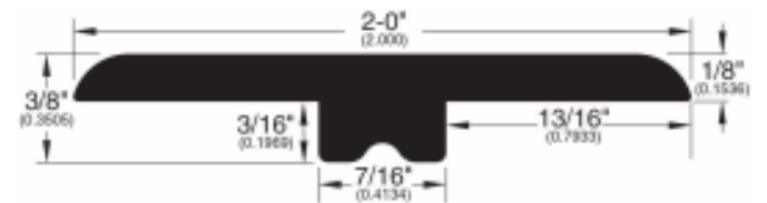
T-Mold (289)
