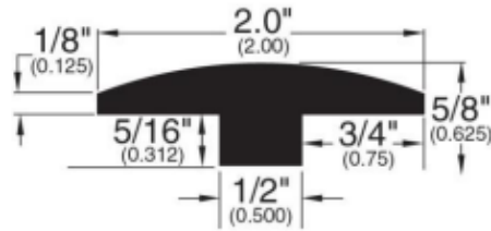
T-Mold (002)
